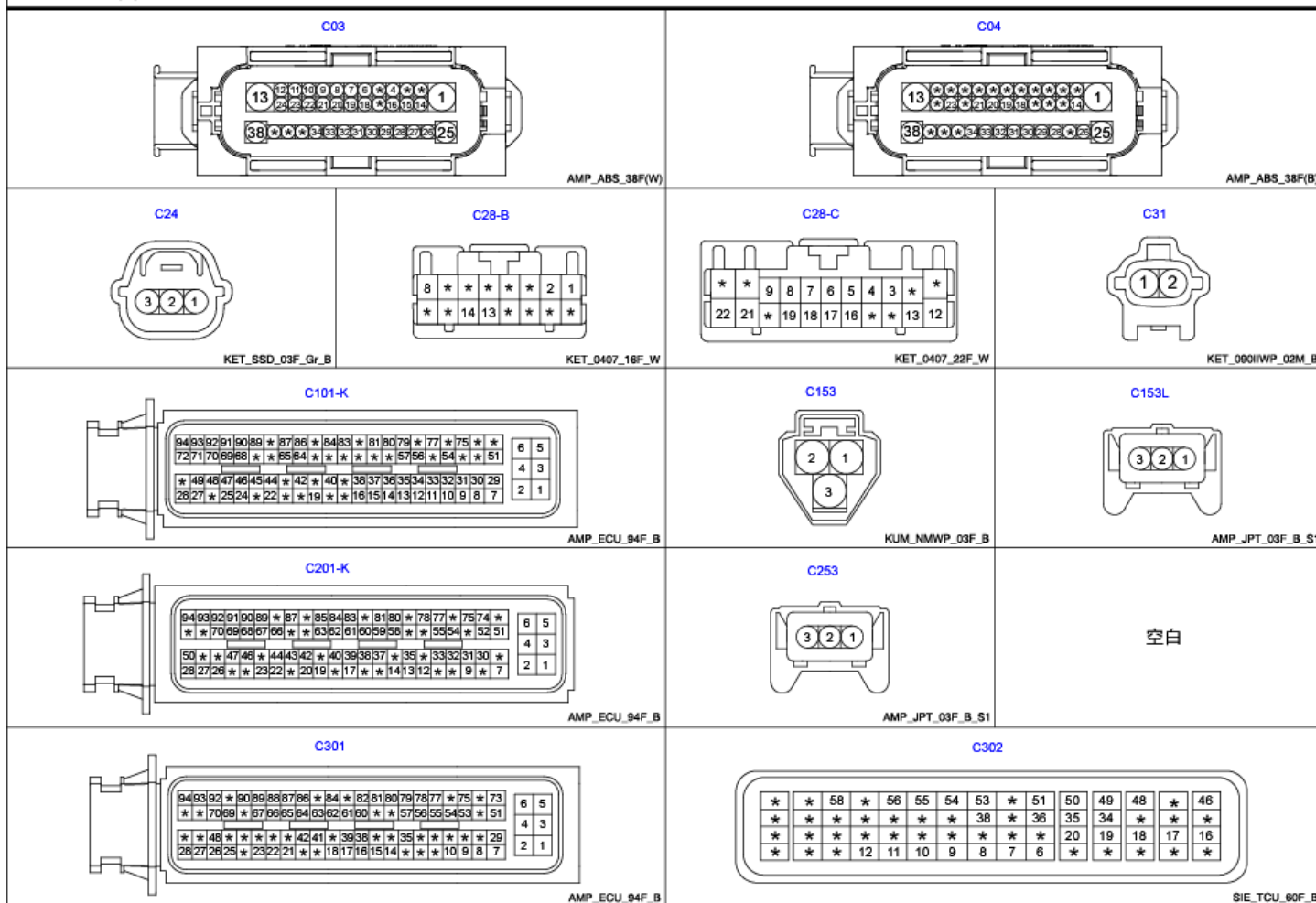
车速系统 (4)
